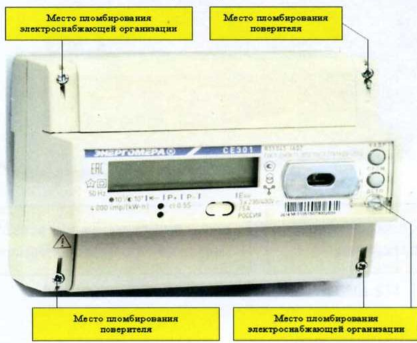
Рисунок 3 – Общий вид счетчика CE301 R33
