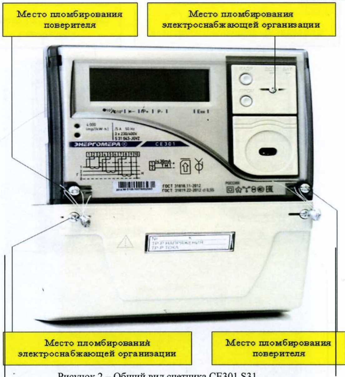
Рисунок 2 – Общий вид счетчика CE301 S31
