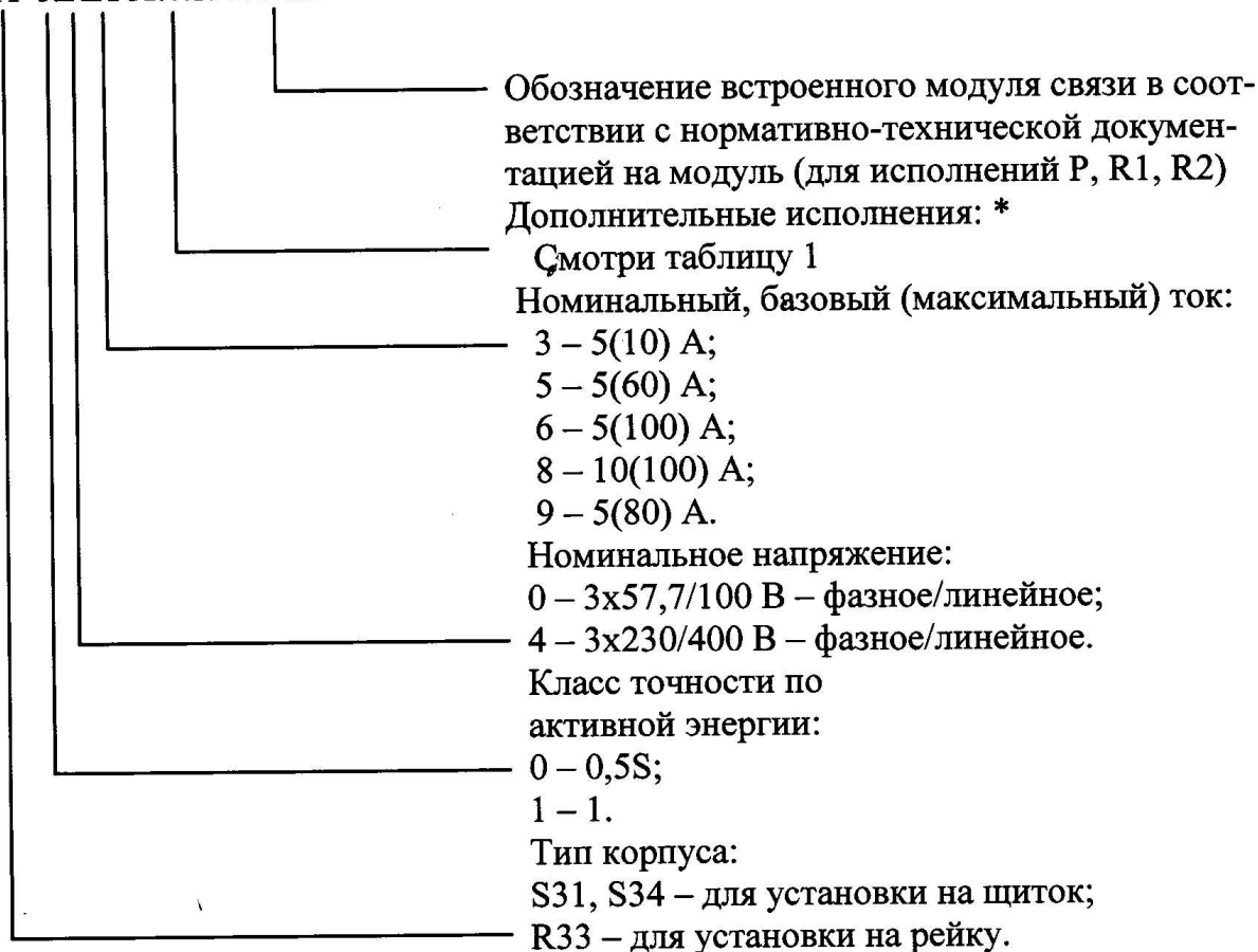
Рисунок 1 - Структура условного обозначения счетчиков
