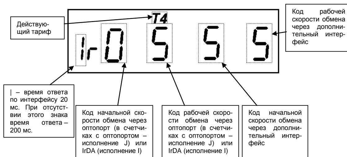
Рисунок 5.16 – Кадр с закодированными скоростями обмена
