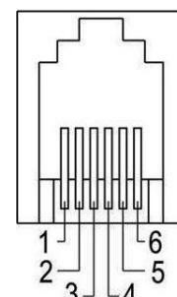
б) обозначение контактов розетки "19" (для исполнений счетчиков с ин-
