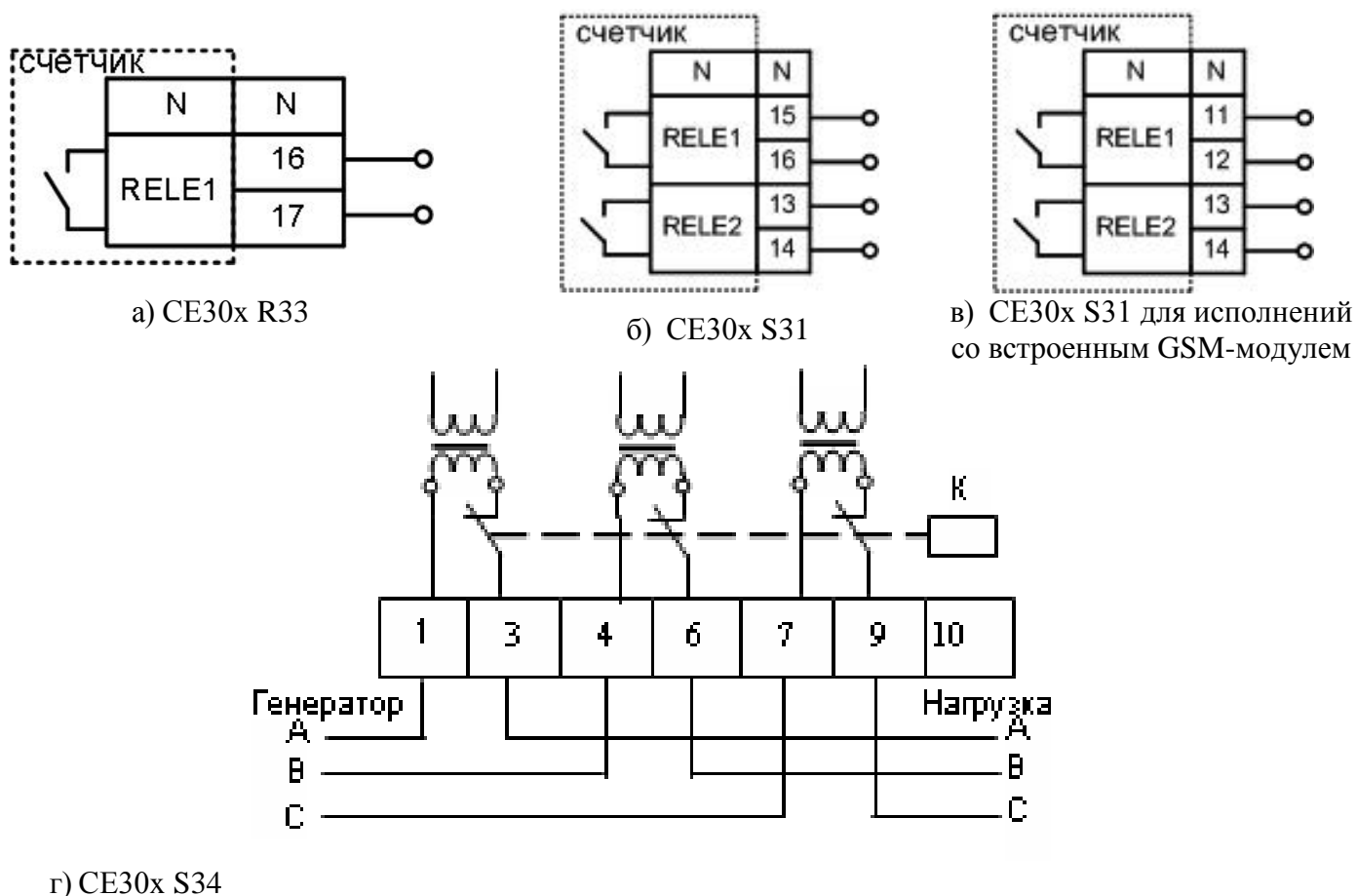
Рисунок 5.5 – Схемы подключения реле
