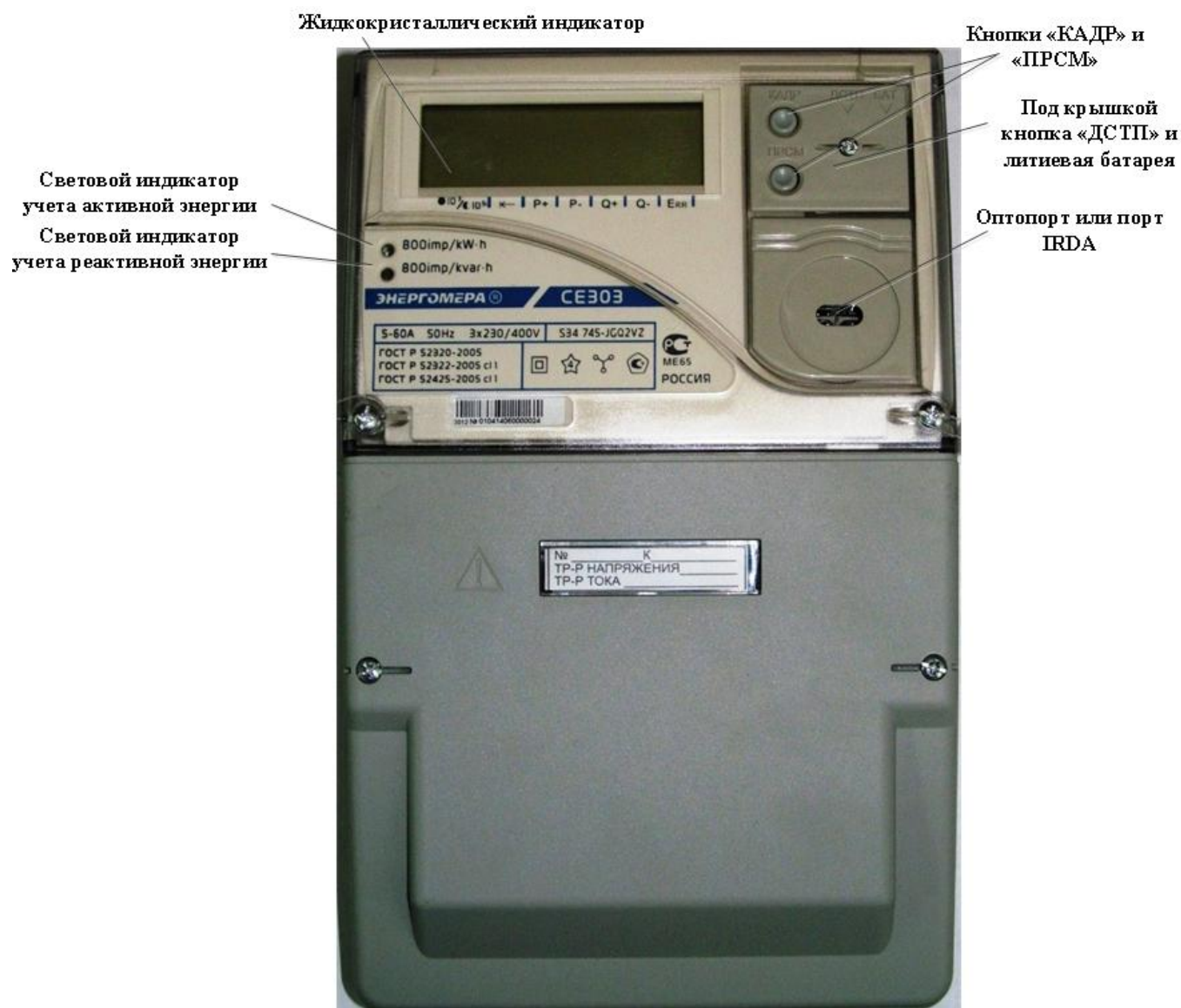
Рисунок 3.2 – Общий вид счетчика
