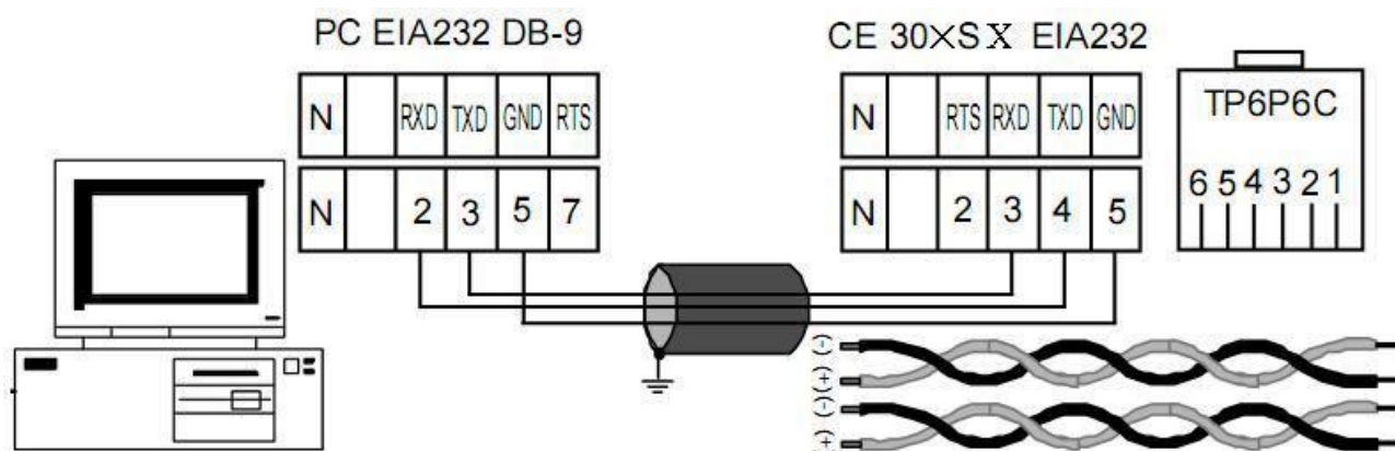
Рисунок 5.9 – Схема подключения счетчика CE30x SX с интерфейсом EIA232 к COM-порту ПЭВМ через кабель
