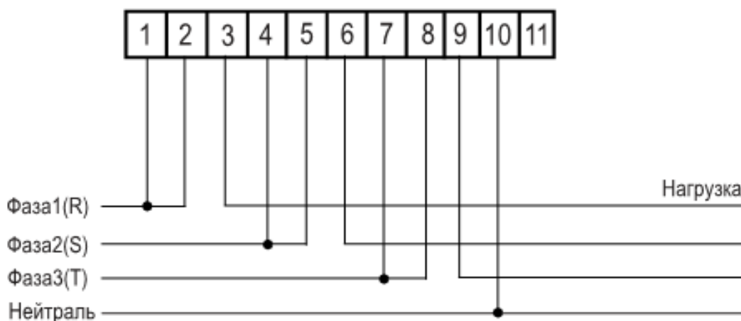
в) Схема включения счетчика СЕ30х 230 В 5(60) А; 5(100) А; 10(100) А
