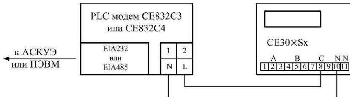
Рисунок 5.12 – Схема подключения счетчика
