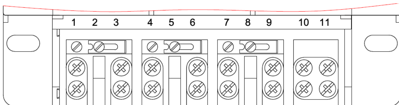
д) – обозначение контактов зажимов счетчика CE303 S31 74X и CE 301 S31 14X
