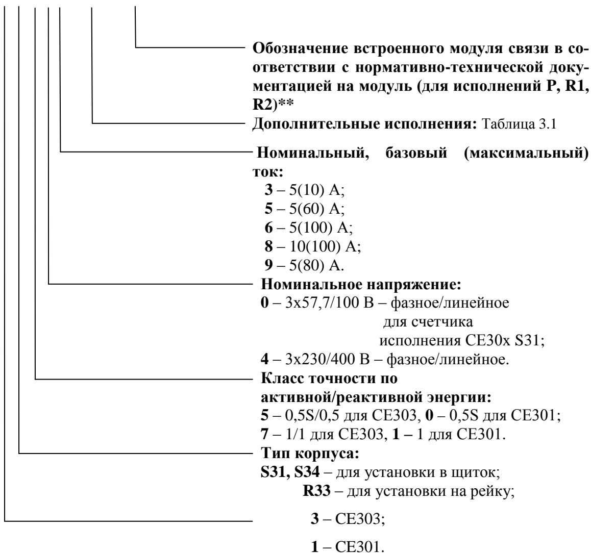
Рисунок 3.1 – Структура условного обозначения
