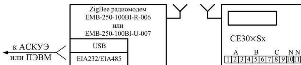
Рисунок 5.11 – Схема подключения счетчика
