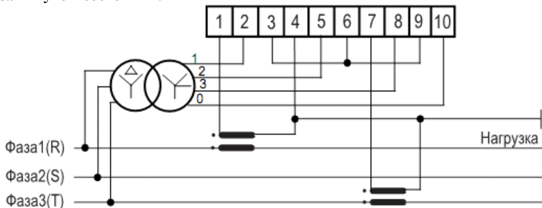
г) Схема включения счетчика СЕ30х S31 57,7 В 5(10) А
