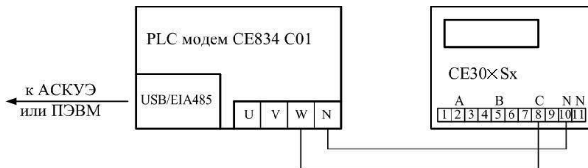
Рисунок 5.13 – Схема подключения счетчика
