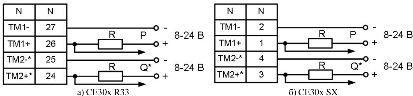
Рисунок 5.4 – Схема подключения импульсных выходов счетчика
