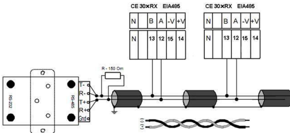
Рисунок 5.7 – Схема подключения счетчика CE30x R33 с интерфейсом EIA485 через внешний адаптер EIA485/EIA232 к COM-порту ПЭВМ
