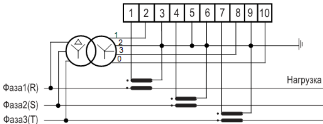
б) Схема включения счетчика СЕ30х S31 57,7 В 5(10) А
