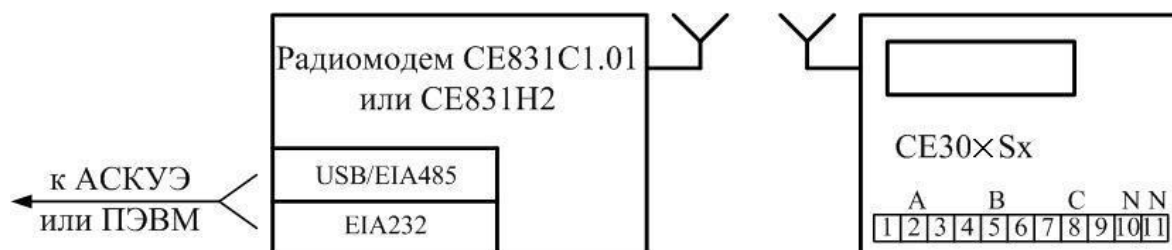
Рисунок 5.10 – Схема подключения счетчика
