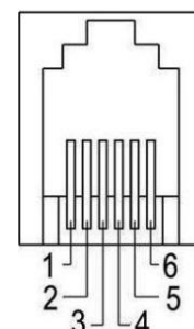
б) обозначение контактов розетки "19" (для исполнений счетчиков с ин-
