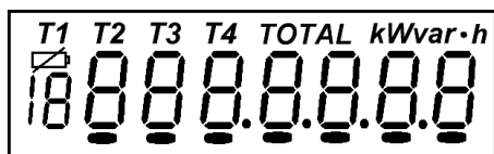
Рисунок 3.4 – Отображаемые символы и знаки на ЖКИ
