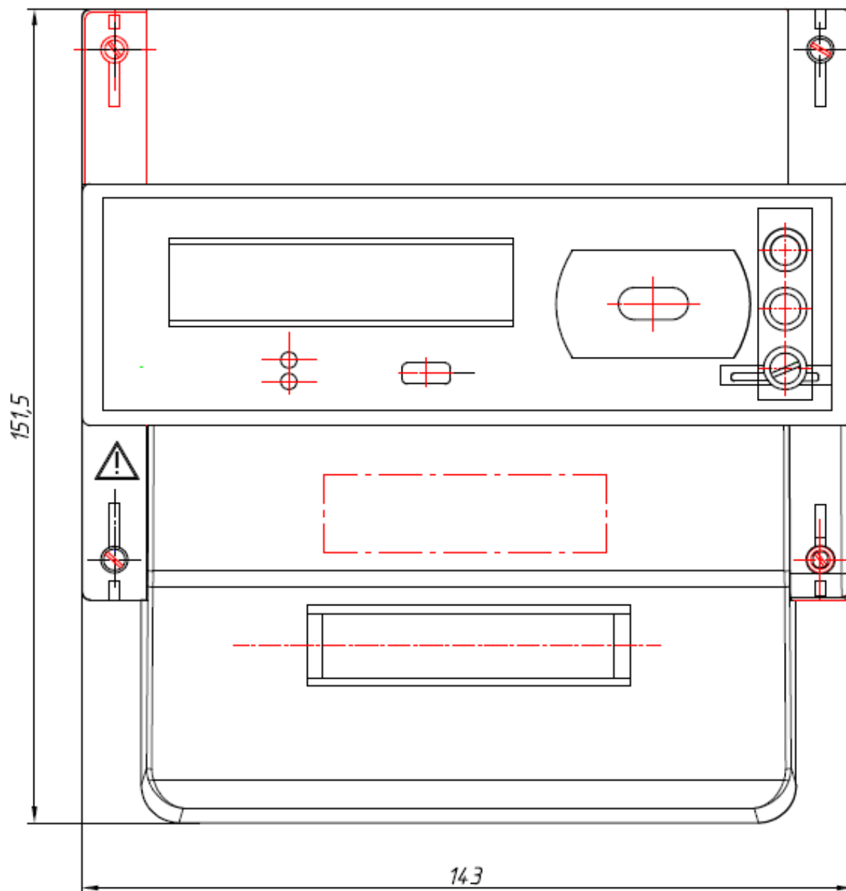
Общий вид счетчика СЕ30х R33
