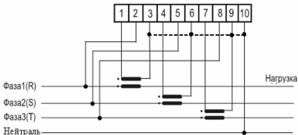
а) Схема включения счетчика СЕ30х 230 В 5(10) А Подключение через три трансформатора тока трехфазная четырехпроводная сеть
