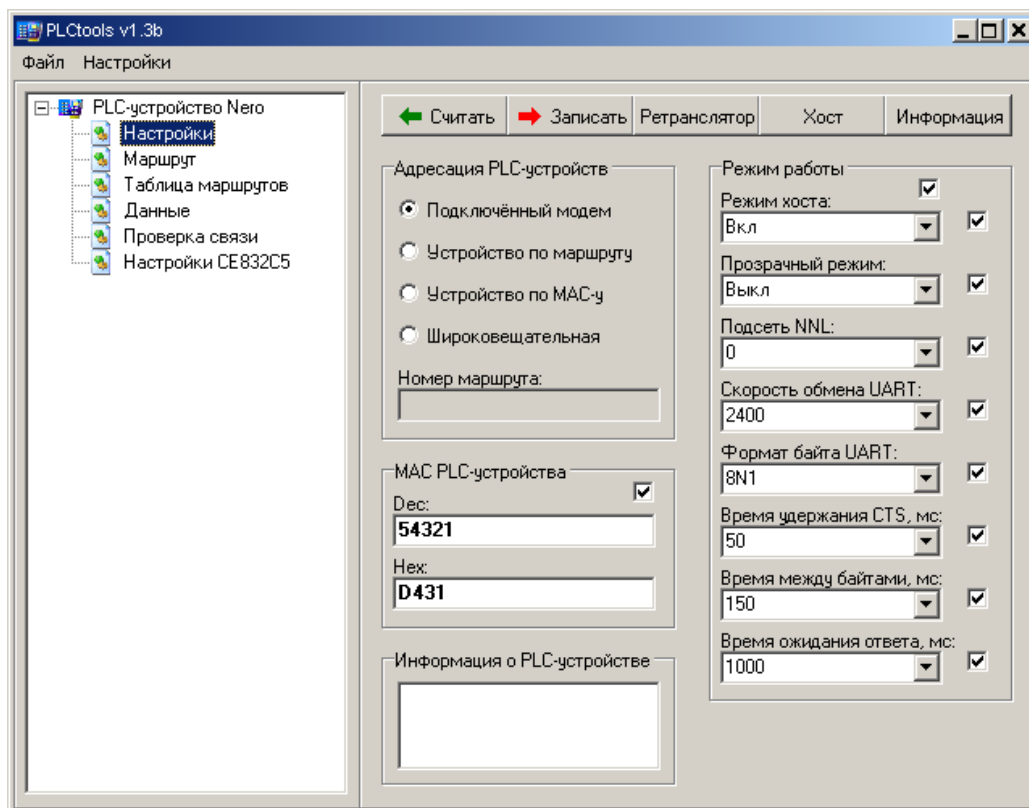
Рисунок 5.23 – Настройки PLC-модема
