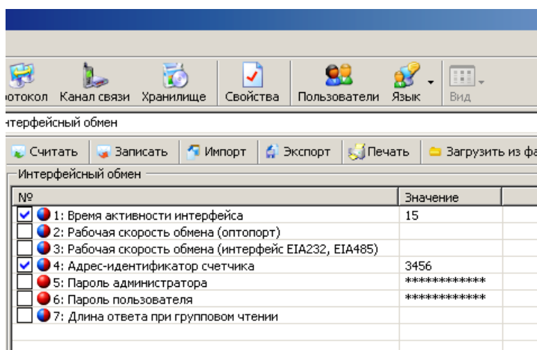
Рисунок 5.17 – Интерфейсный обмен
